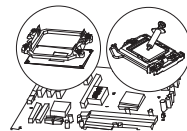
步骤2 拆除AMD主板上原来的塑料挂扣, 均匀涂抹导热硅脂
